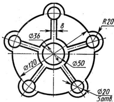
Вариант 1 Фланец
