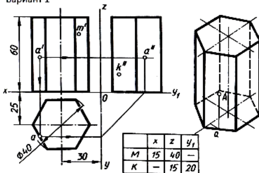
Вариант 1
