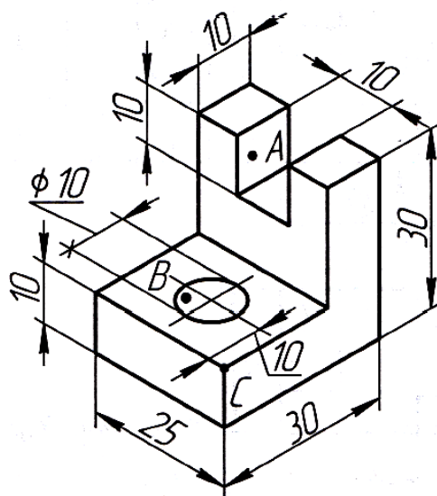
Вариант 2
