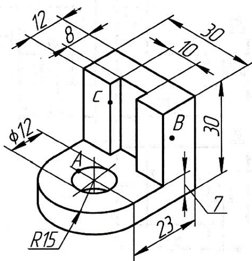
Вариант 1
