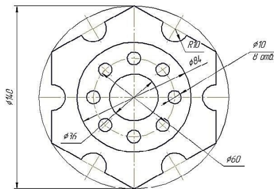
Вариант 1 Фланец
