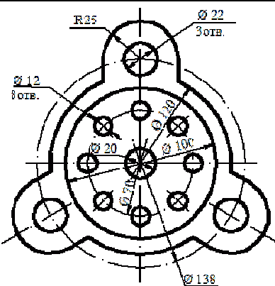
Вариант 3 Фланец
