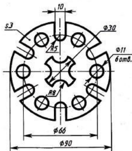
Вариант 6
